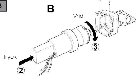
Bild 2- Pumpen skall inte skruvas direkt på skrovet
