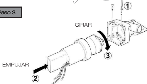
dibujo 3- No atornille la bomba directamente al casco
