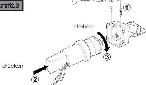
Abb 3. Die Pumpe darf nicht direkt an den Rumpf geschraubt werden
