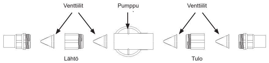
Kuva 2 Pumpun pää
