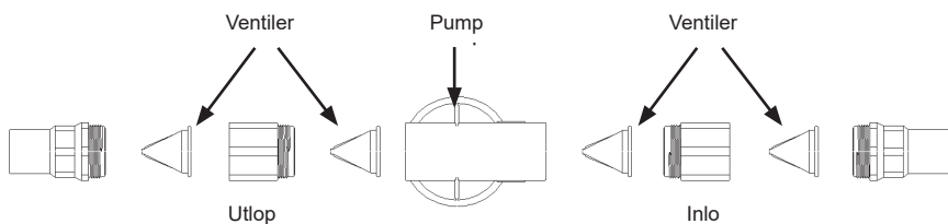
Fig. 2 Pumphuvud
