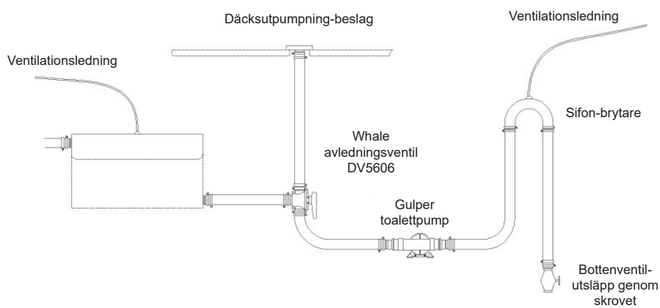
Fig. 4 Typisk utpumpning
