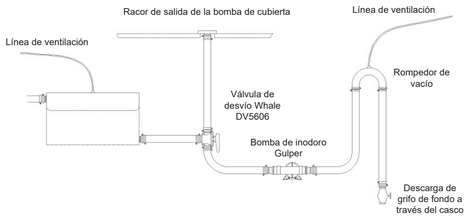
Fig. 4 Bombeo típico
