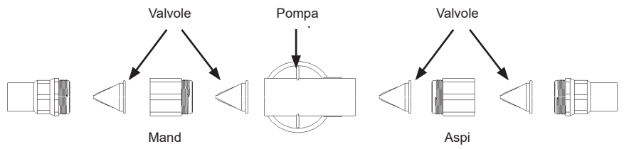
Fig. 2 Testata
