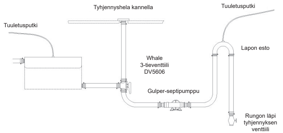
Kuva 4 Tyypillinen tyhjennuspumppaus
