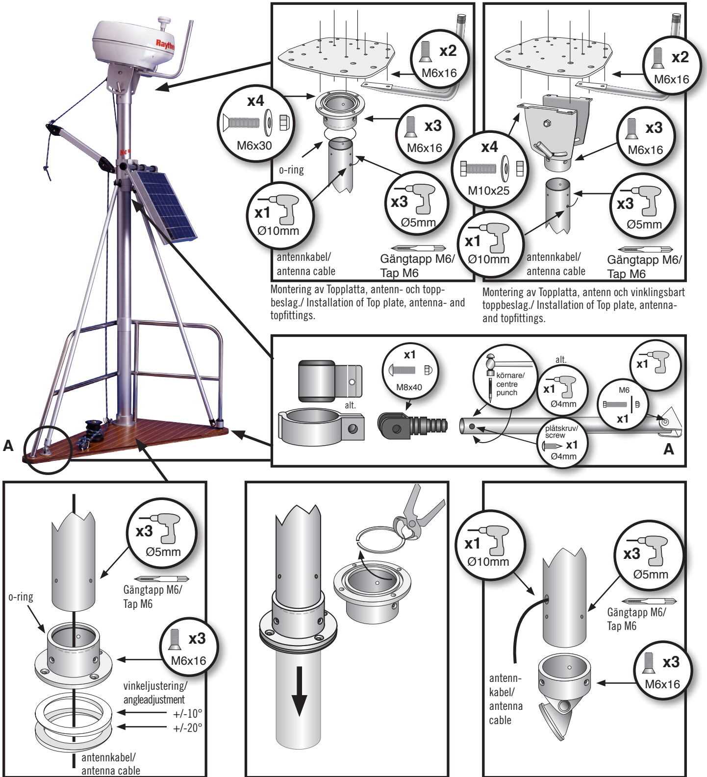
Montering av Däcksfäste./ Installation of deckmounting.
